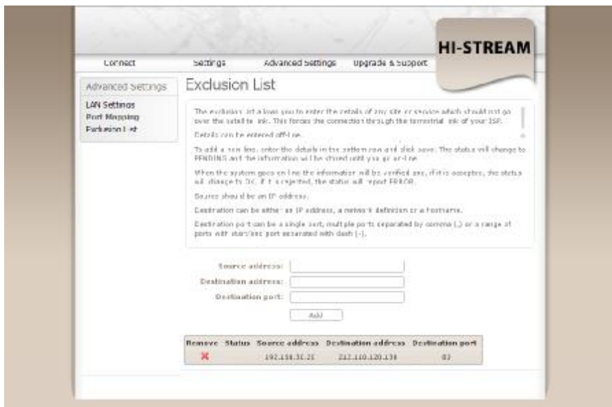
Рисунок 14: Список исключений
