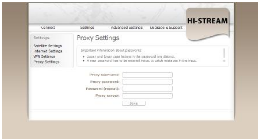
Рисунок 11: Настройки прокси
