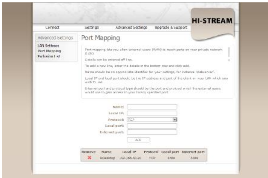
Рисунок 13: Отображение портов
